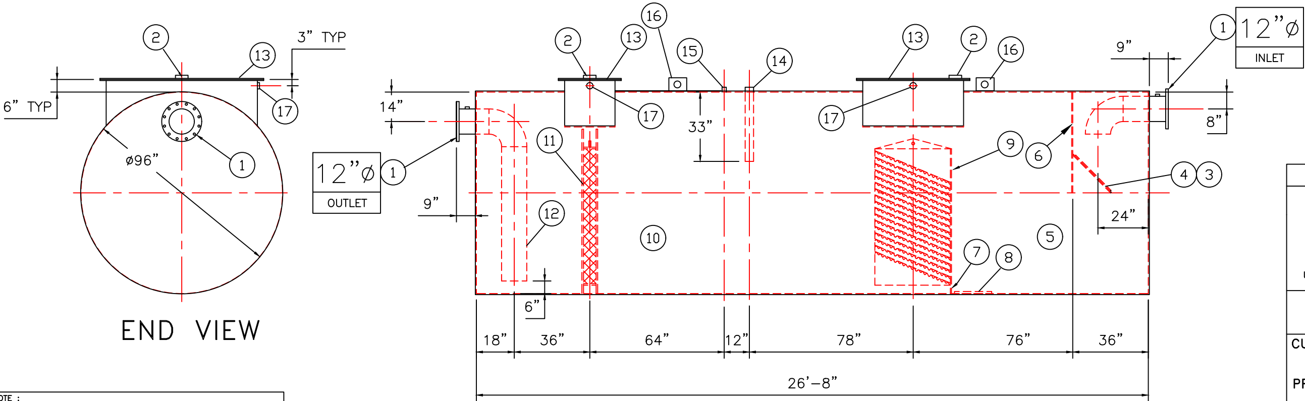
ELEVATION
