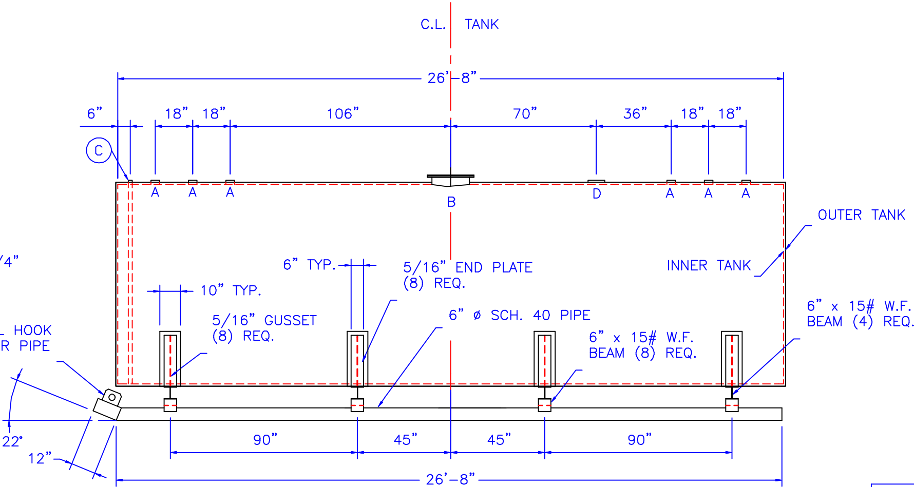
ELEVATION
