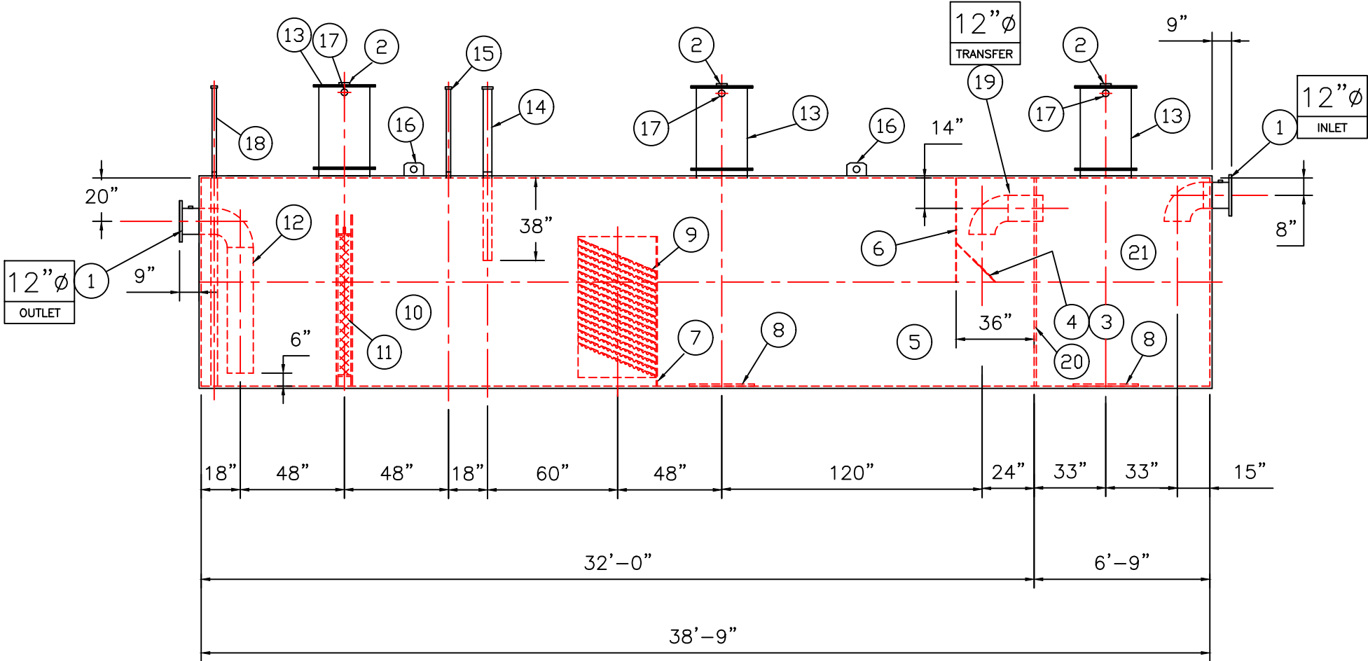
ELEVATION
