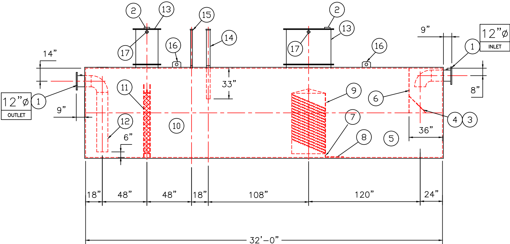
ELEVATION
