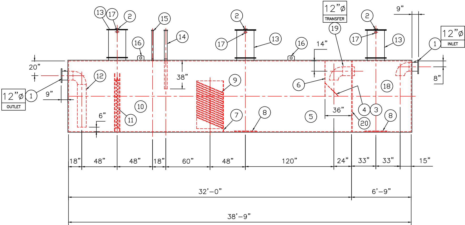
ELEVATION
