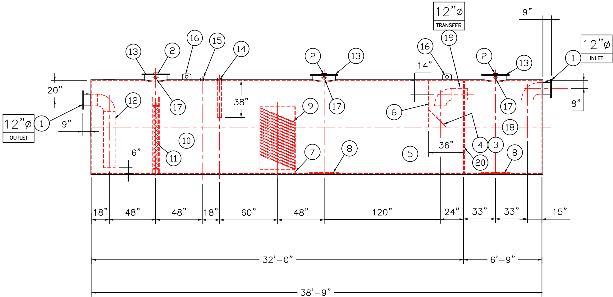
ELEVATION
