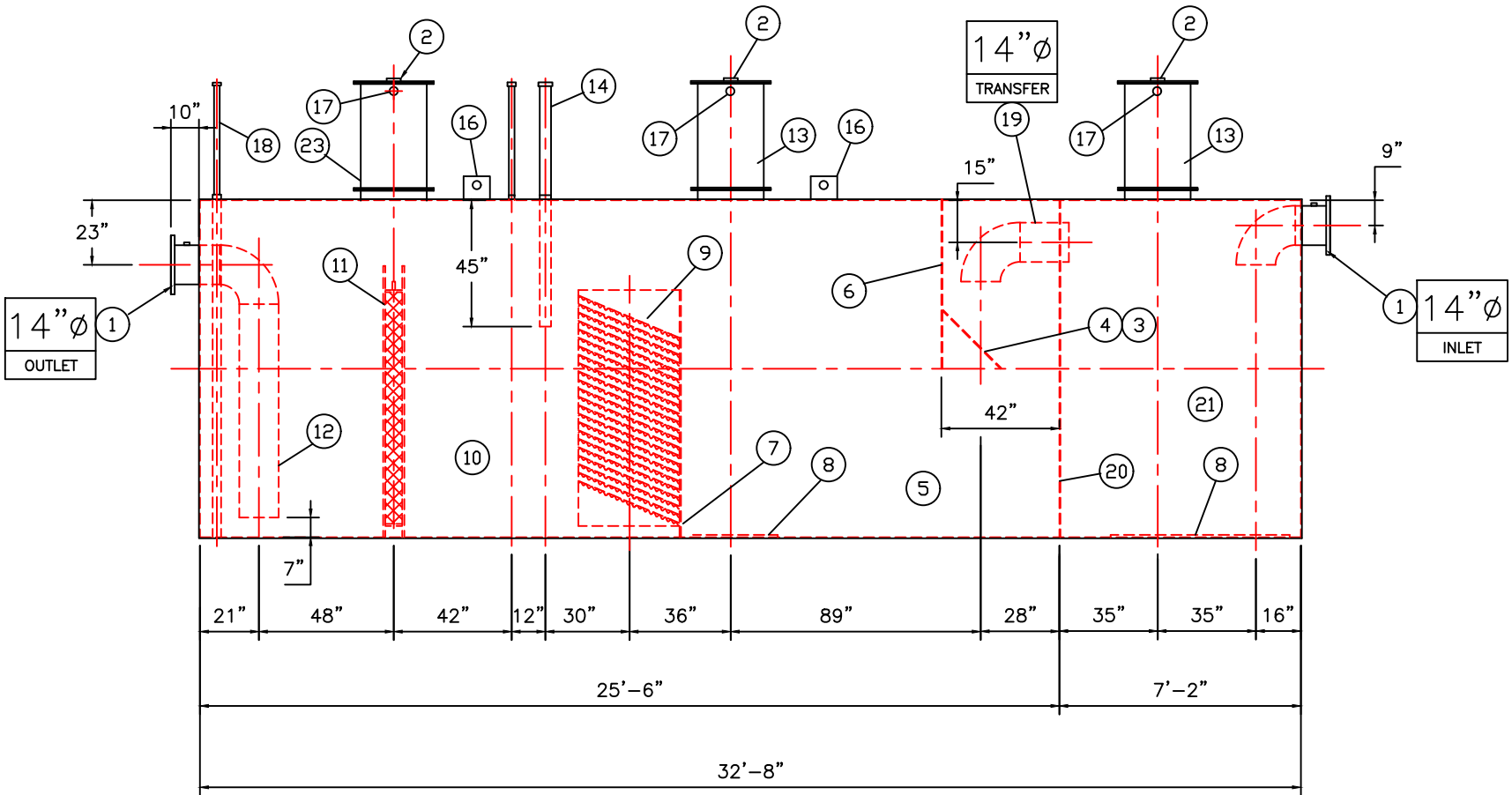
ELEVATION
