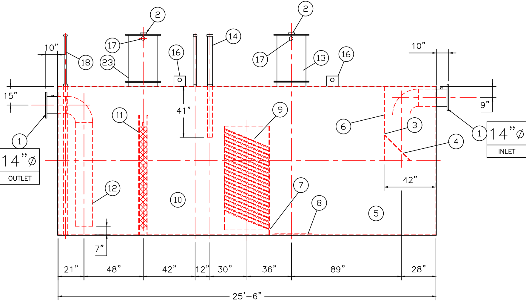
ELEVATION
