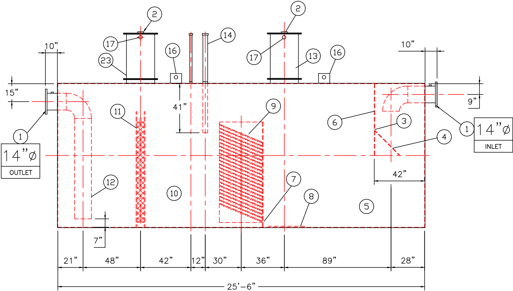
ELEVATION
