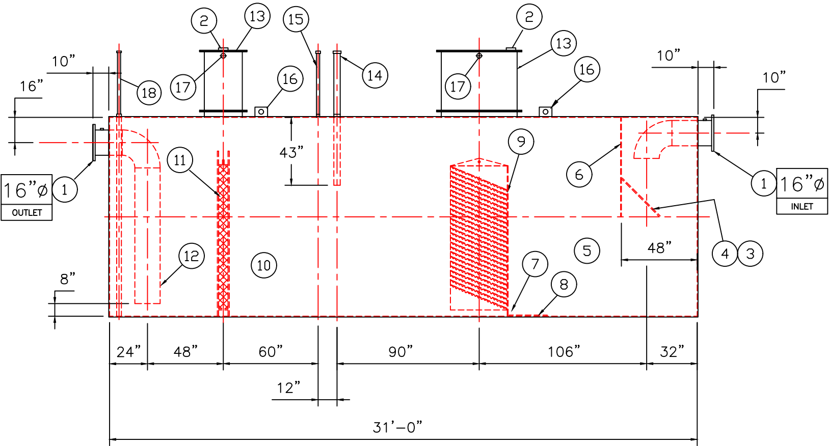
ELEVATION
