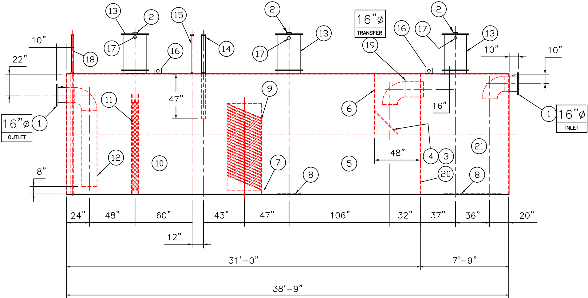
ELEVATION
