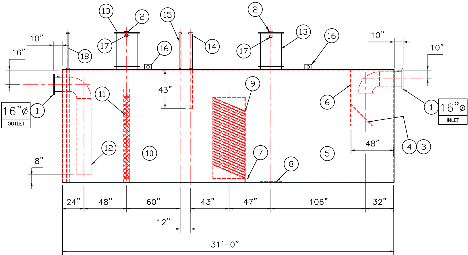
ELEVATION
