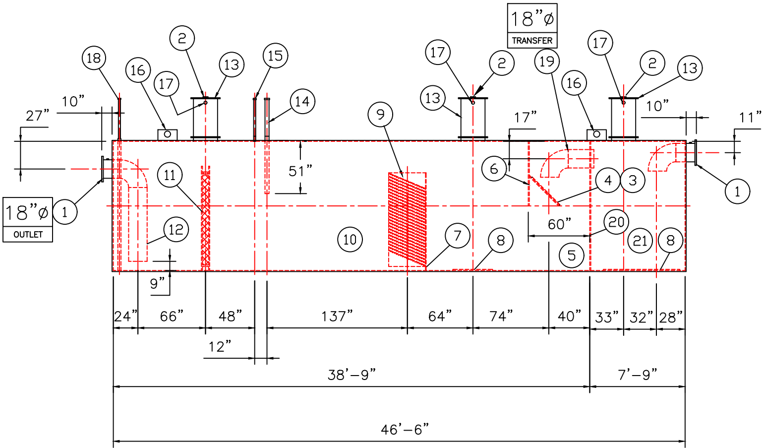
ELEVATION
