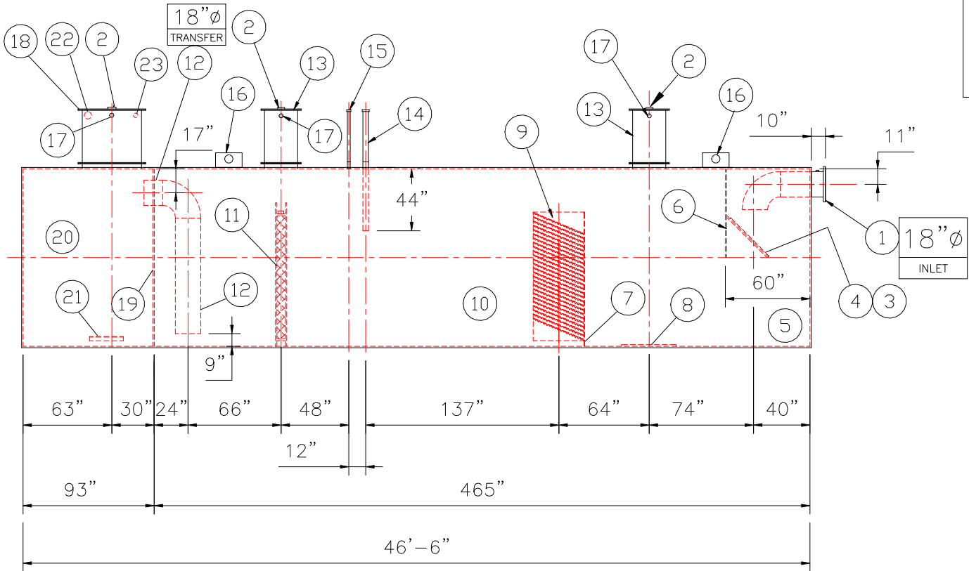
ELEVATION
