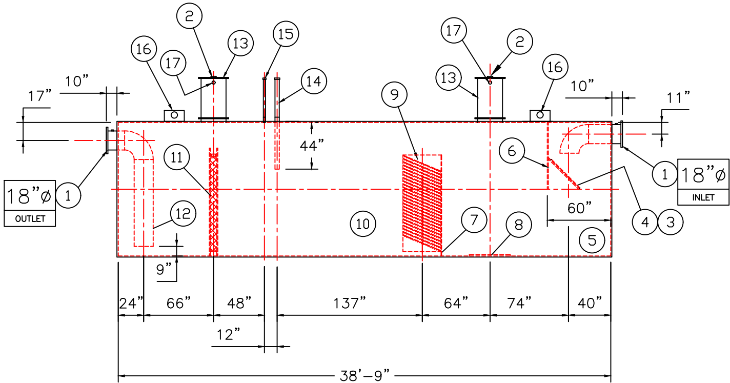
ELEVATION
