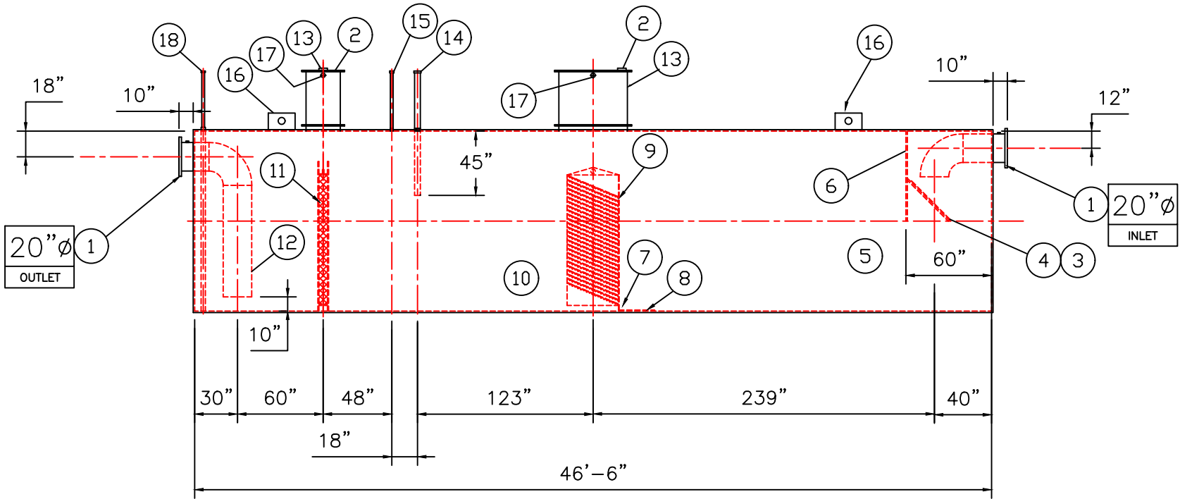
ELEVATION
