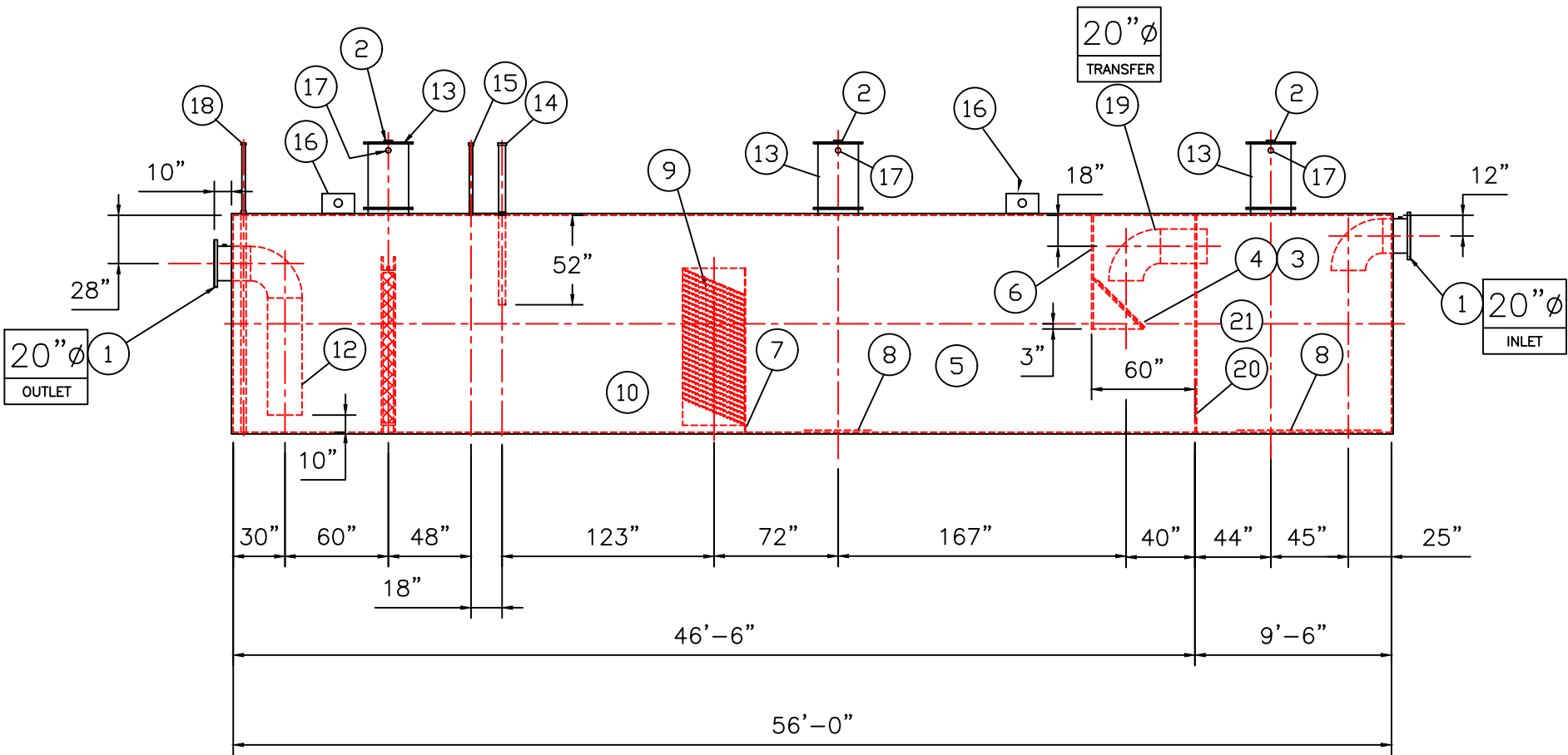
ELEVATION
