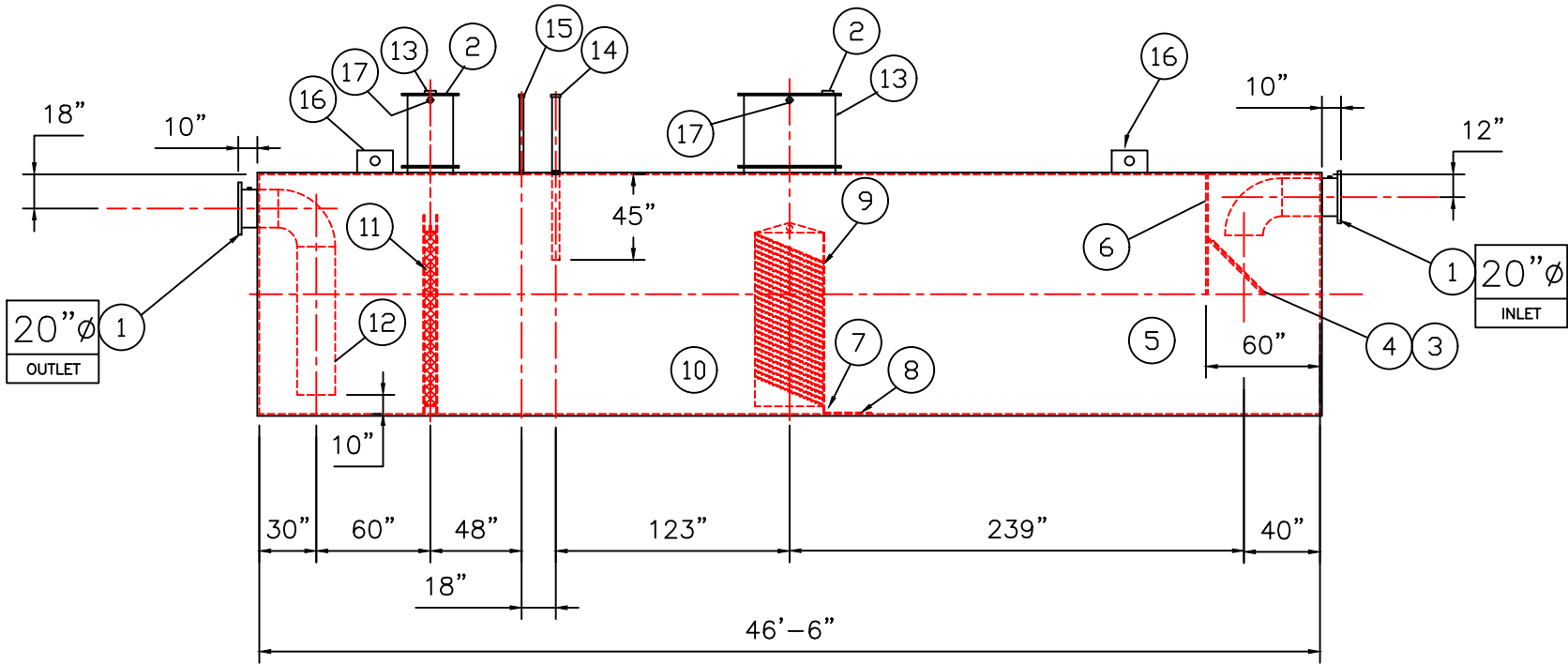
ELEVATION
