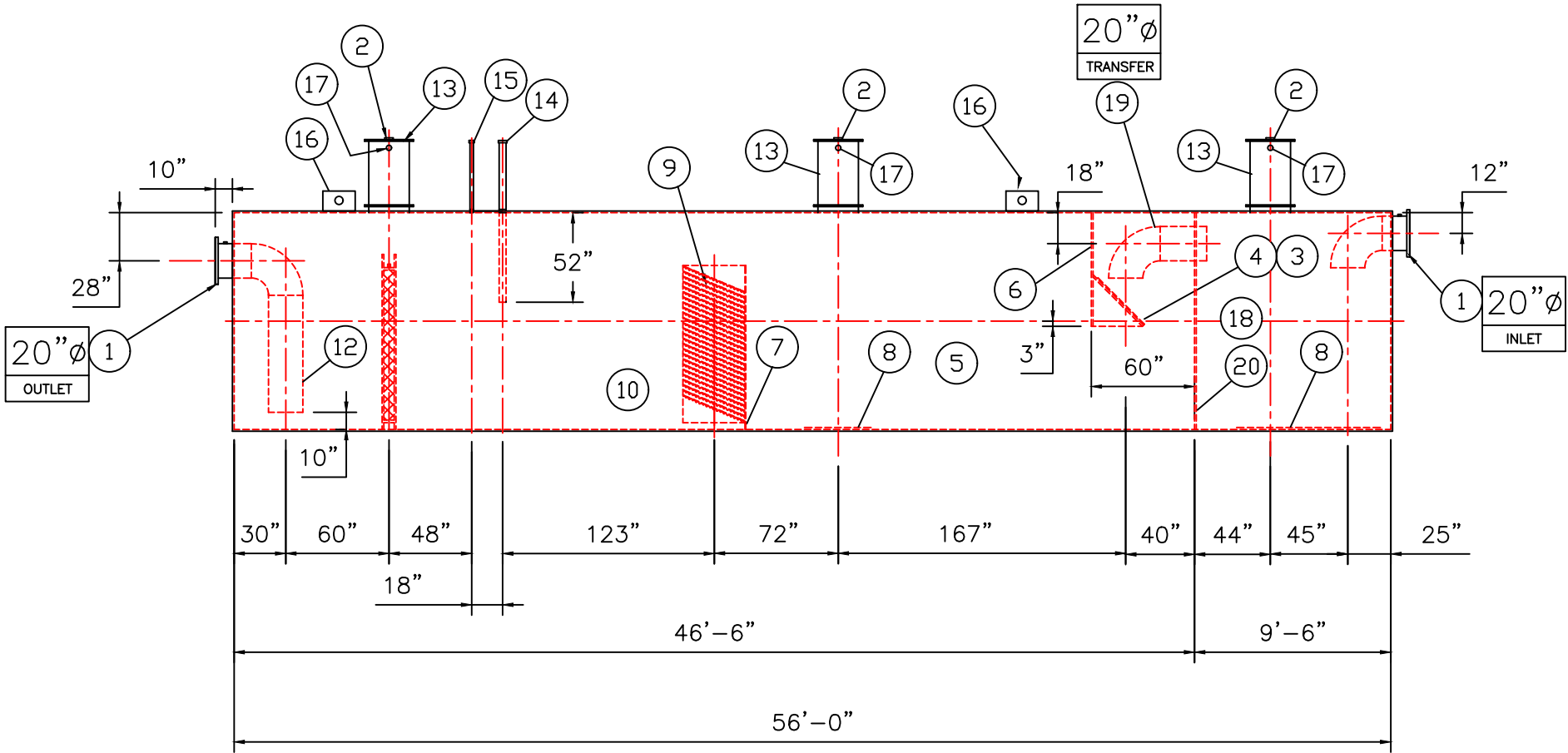
ELEVATION
