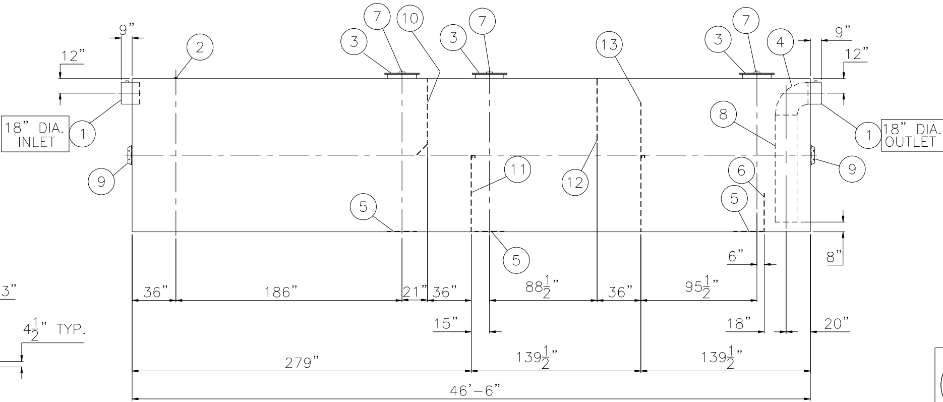
ELEVATION
