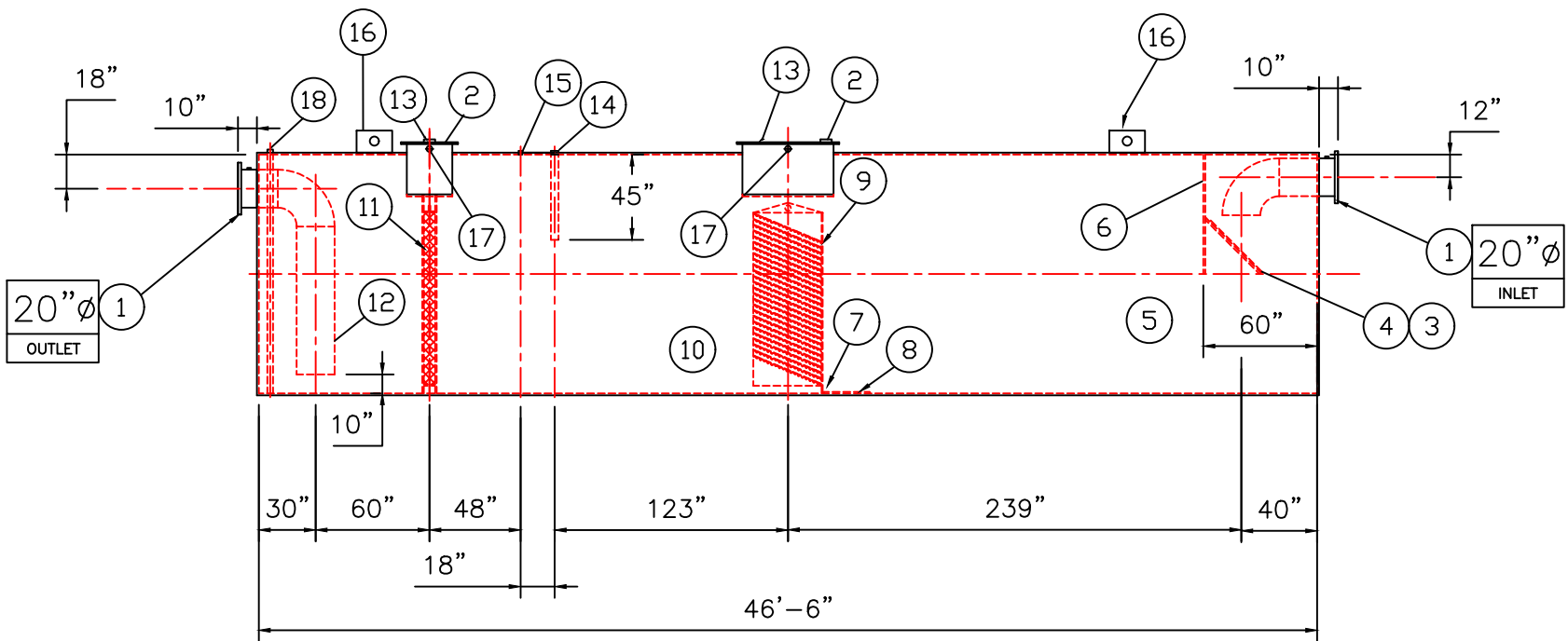
ELEVATION
