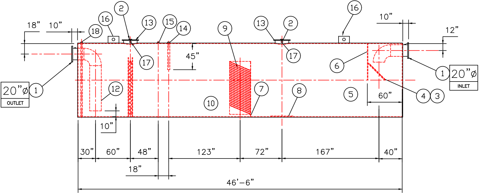
ELEVATION
