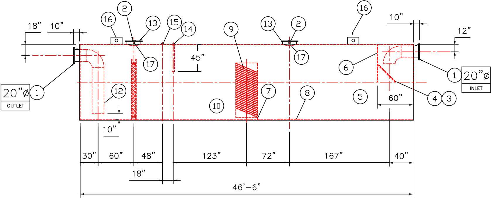
ELEVATION
