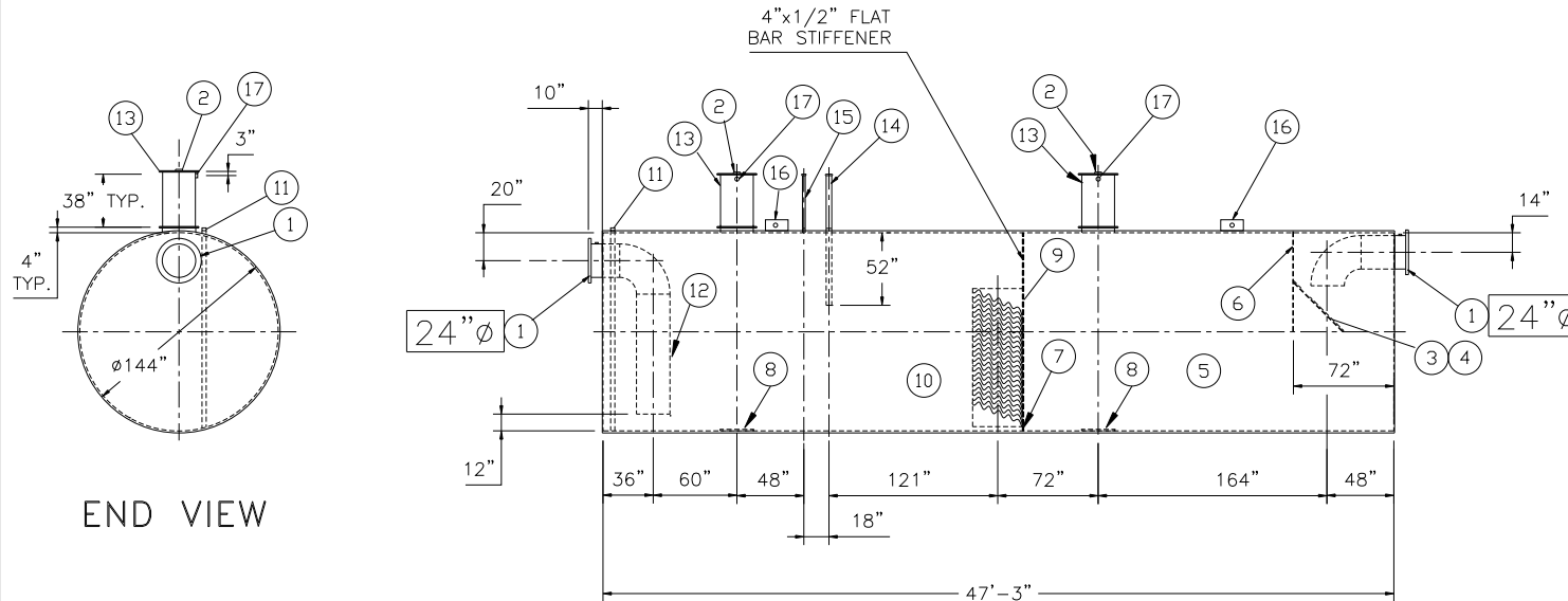
ELEVATION
