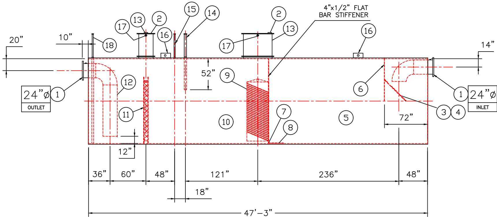
ELEVATION
