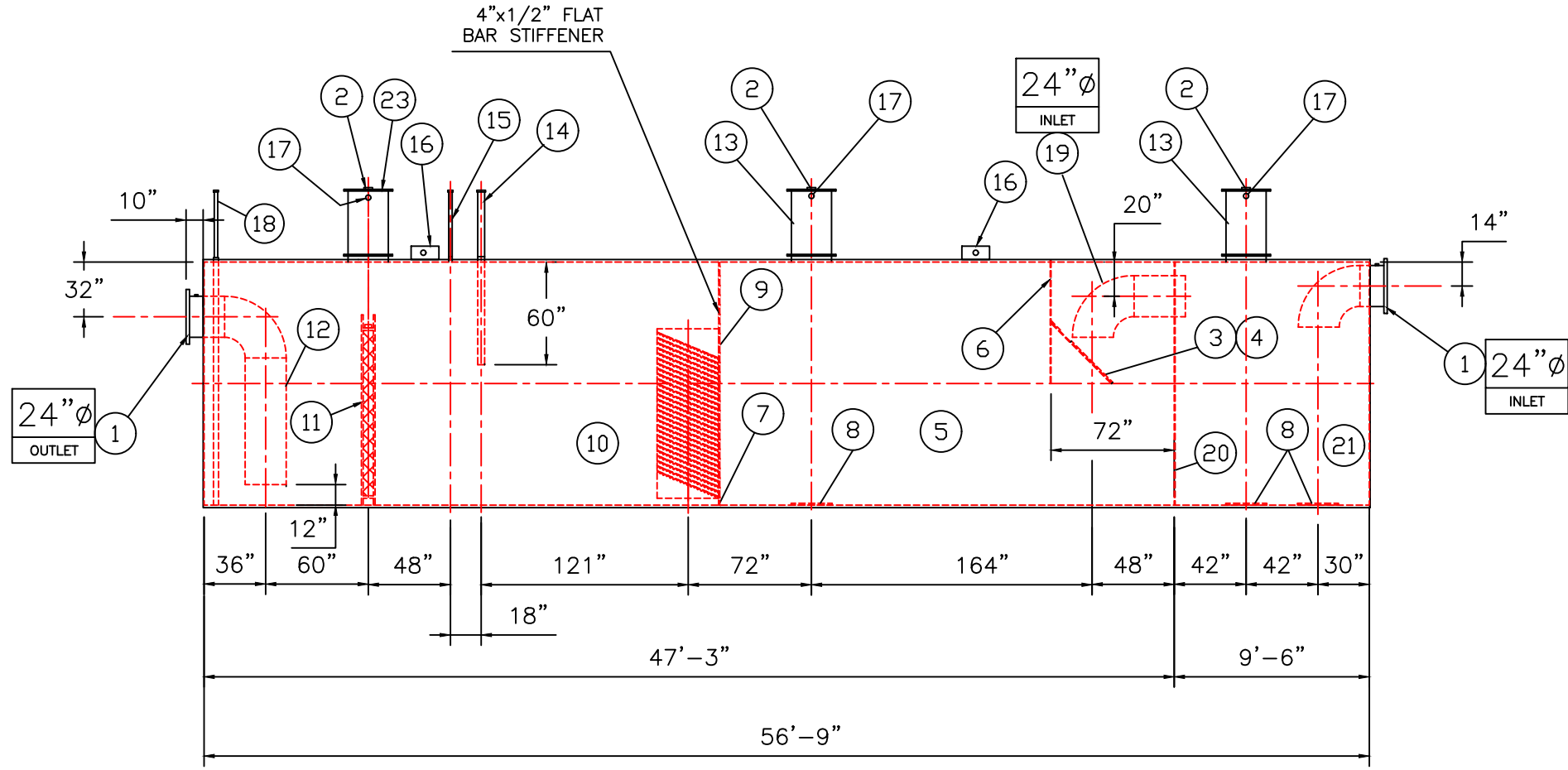
ELEVATION
