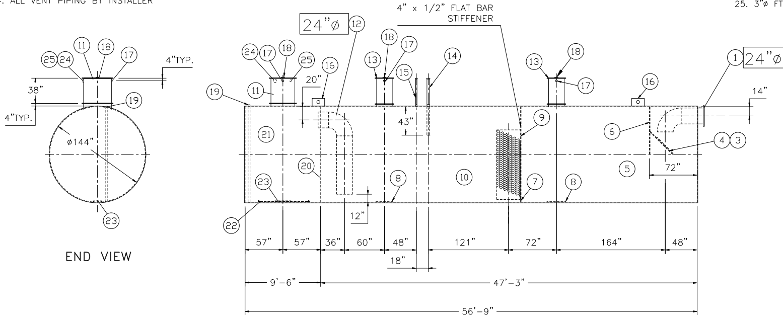
ELEVATION
