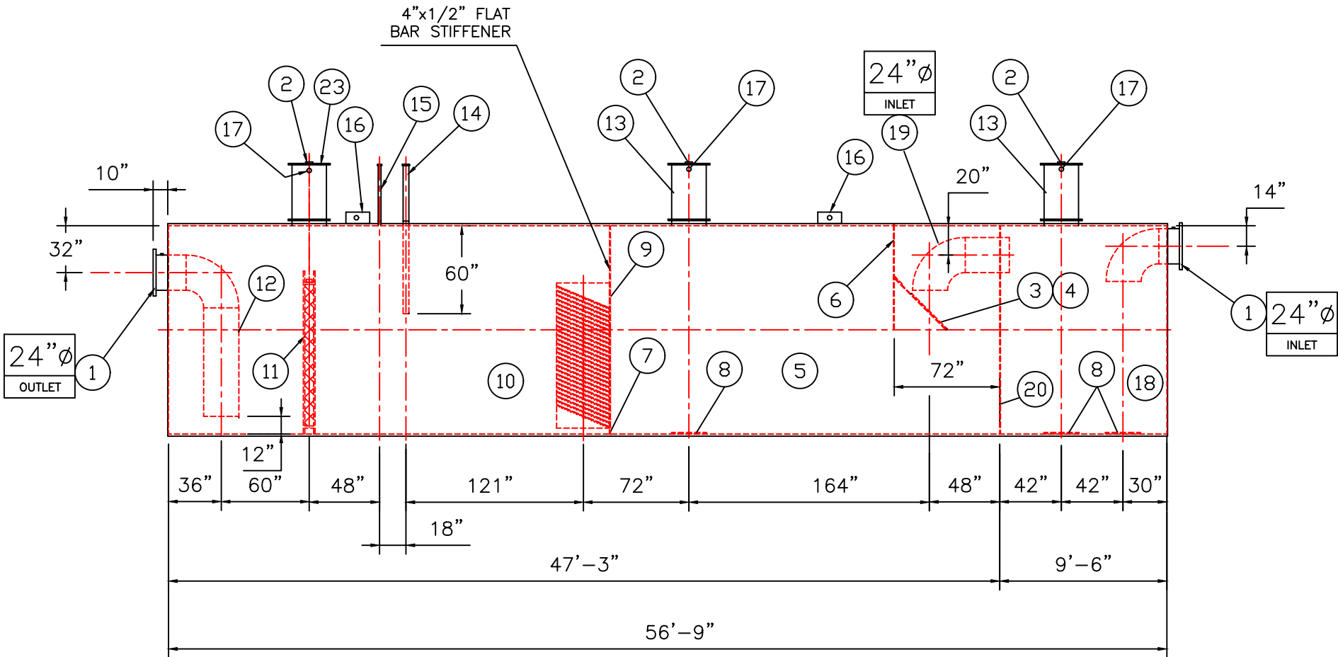
ELEVATION
