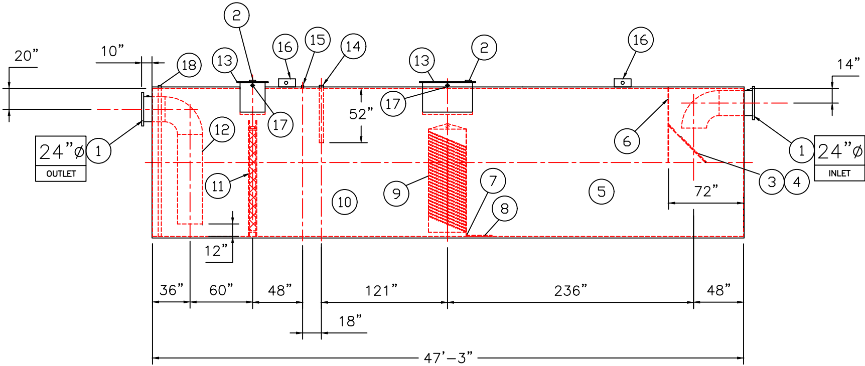
ELEVATION
