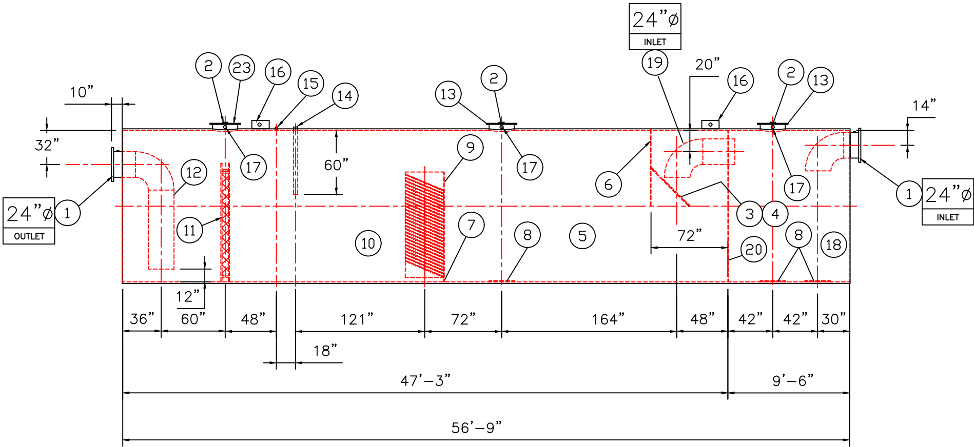
ELEVATION
