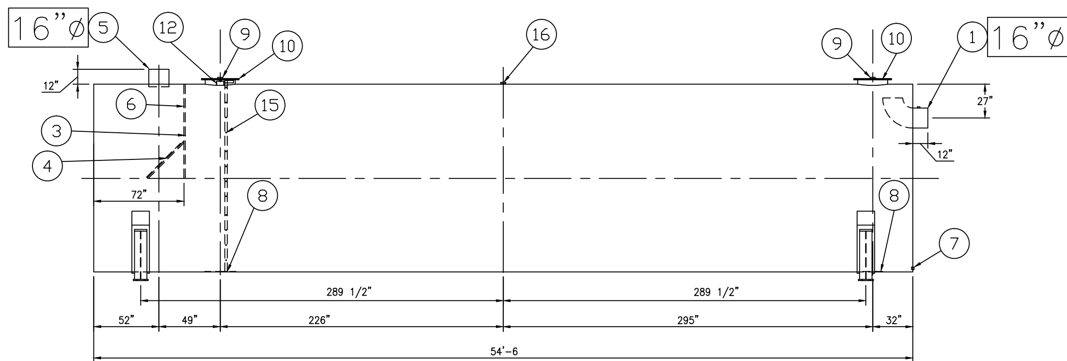
ELEVATION
