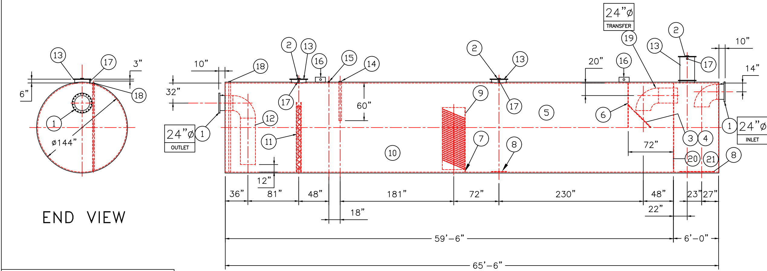
ELEVATION
