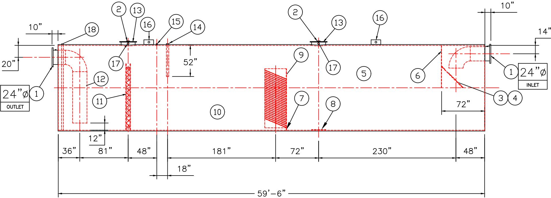
ELEVATION
