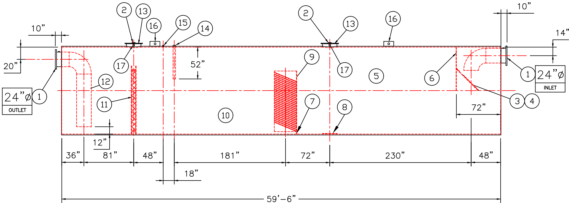
ELEVATION
