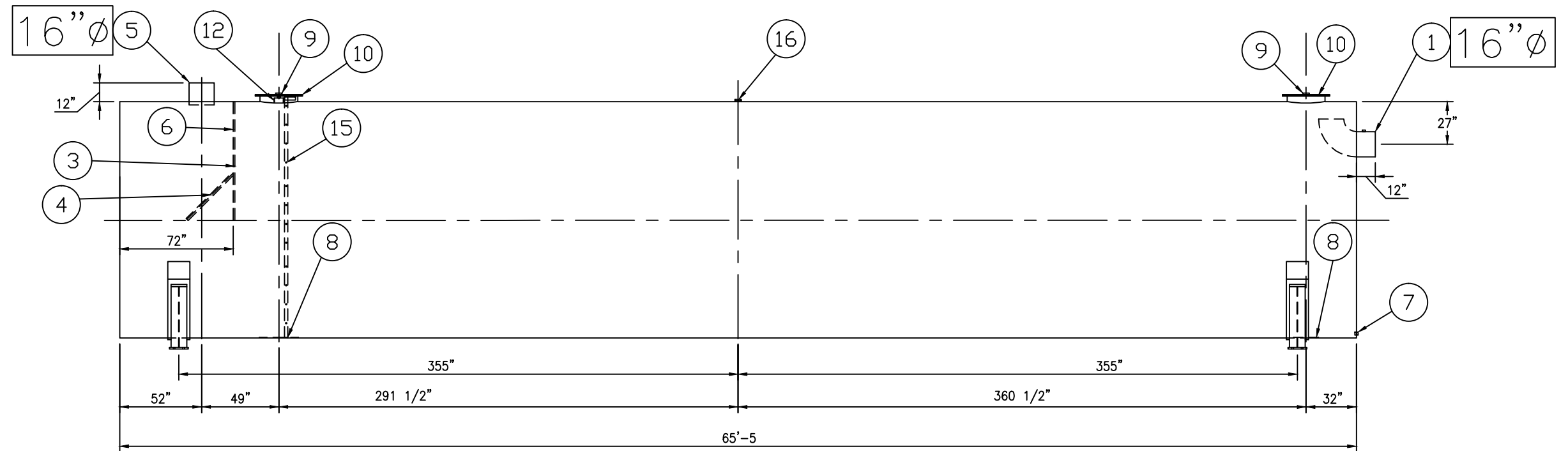
ELEVATION
