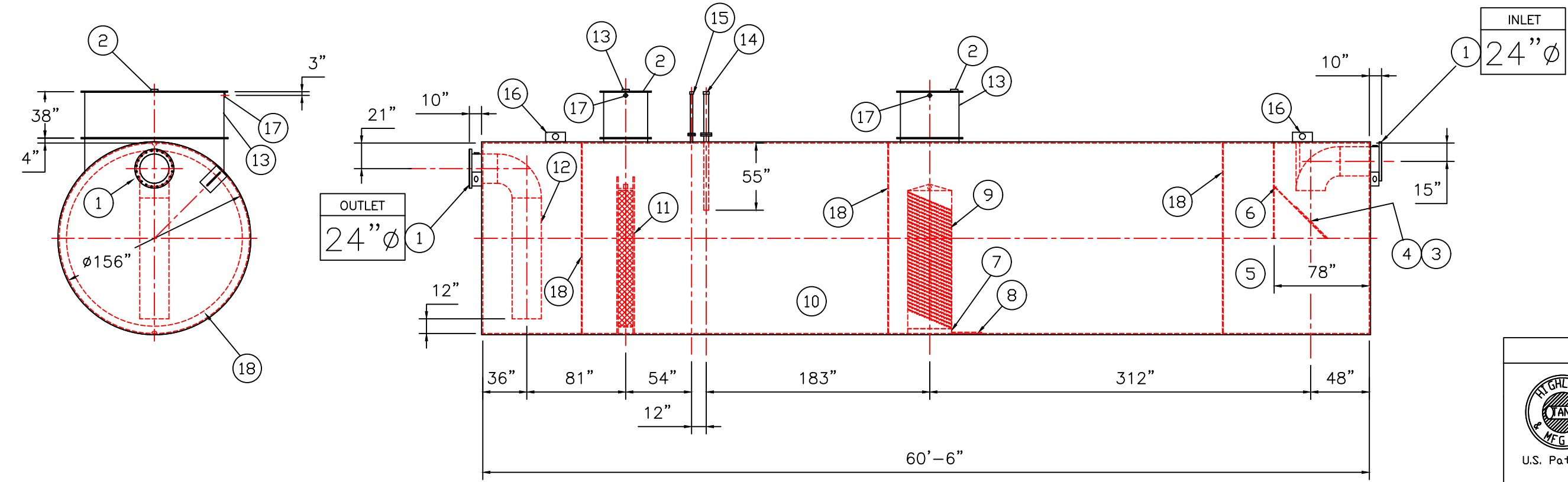
ELEVATION
