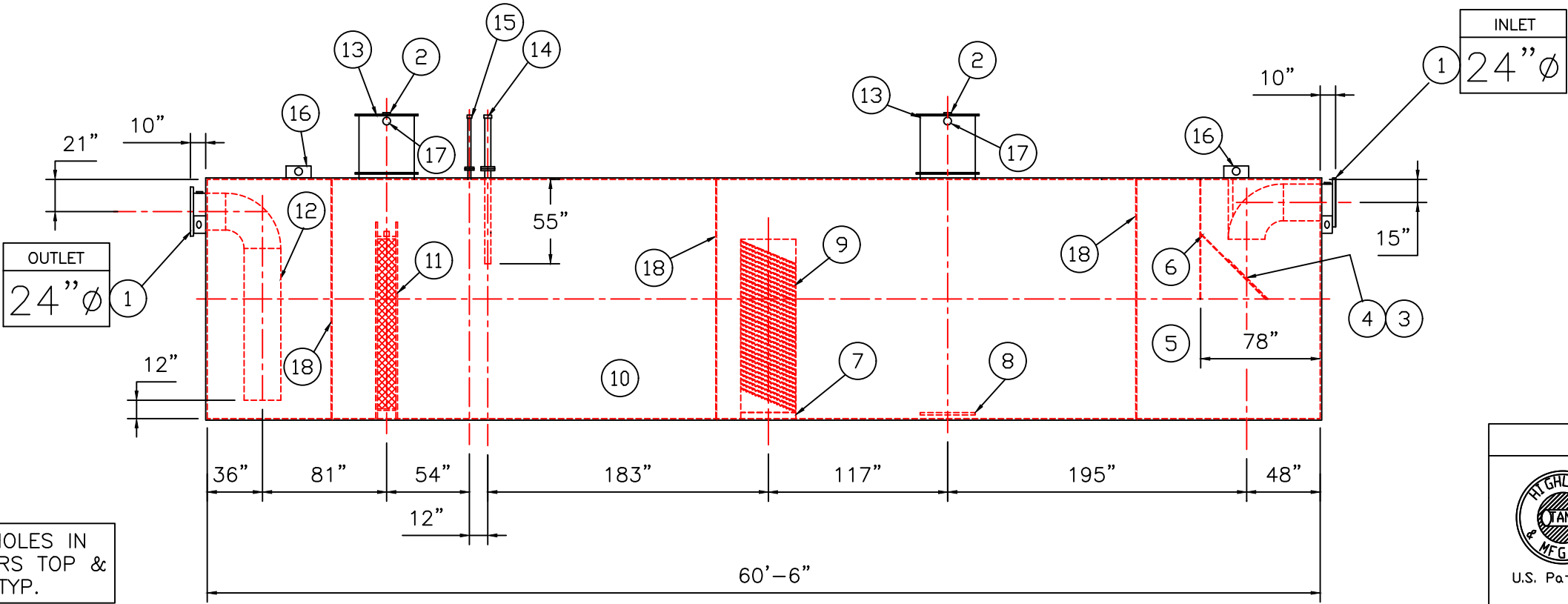
ELEVATION
