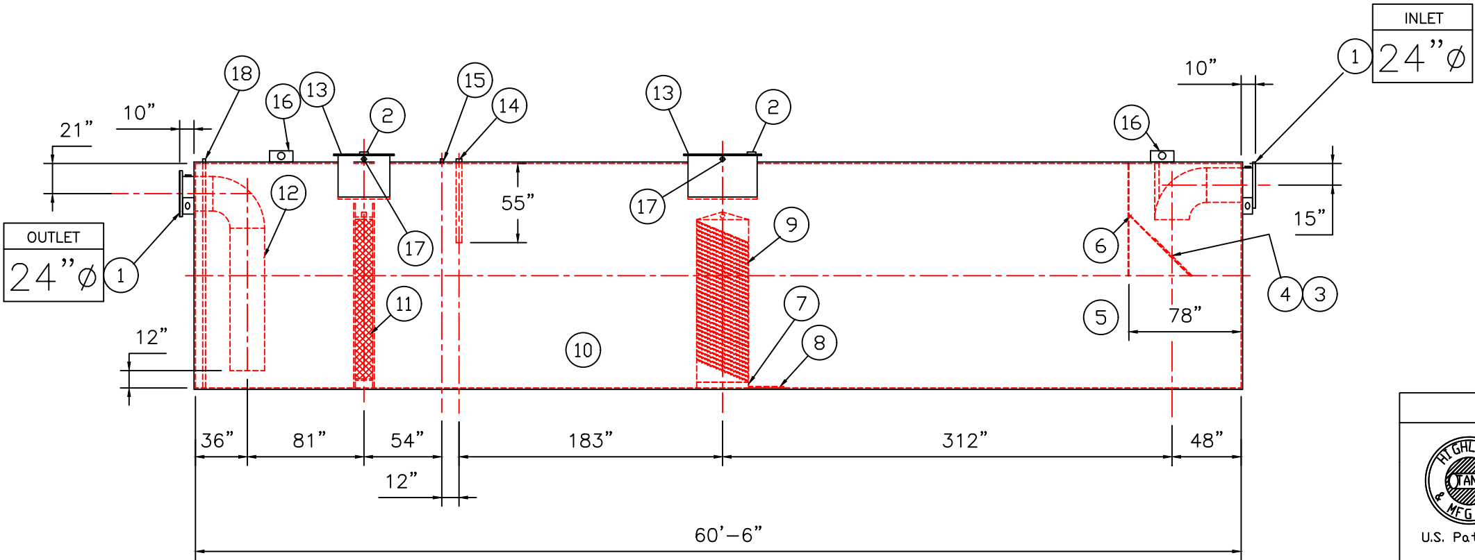
ELEVATION
