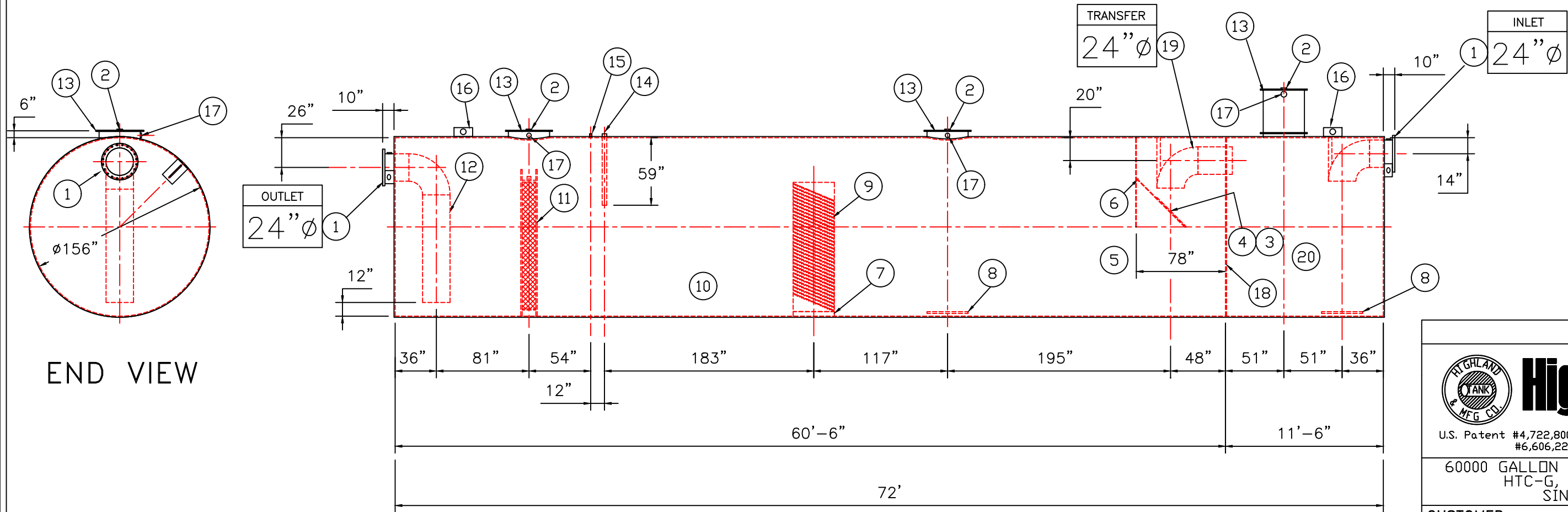
ELEVATION
